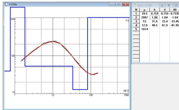
Gambar 3. Titik Pengukuran Geolistrik 1 (T-01)
