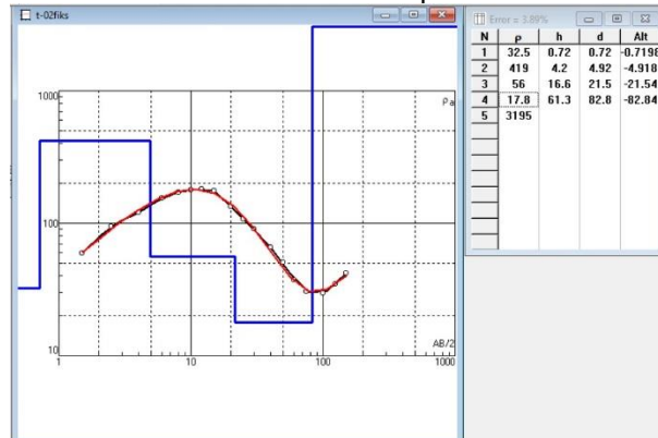
Gambar 4. Titik Pengukuran Geolistrik 2 (T-02)
